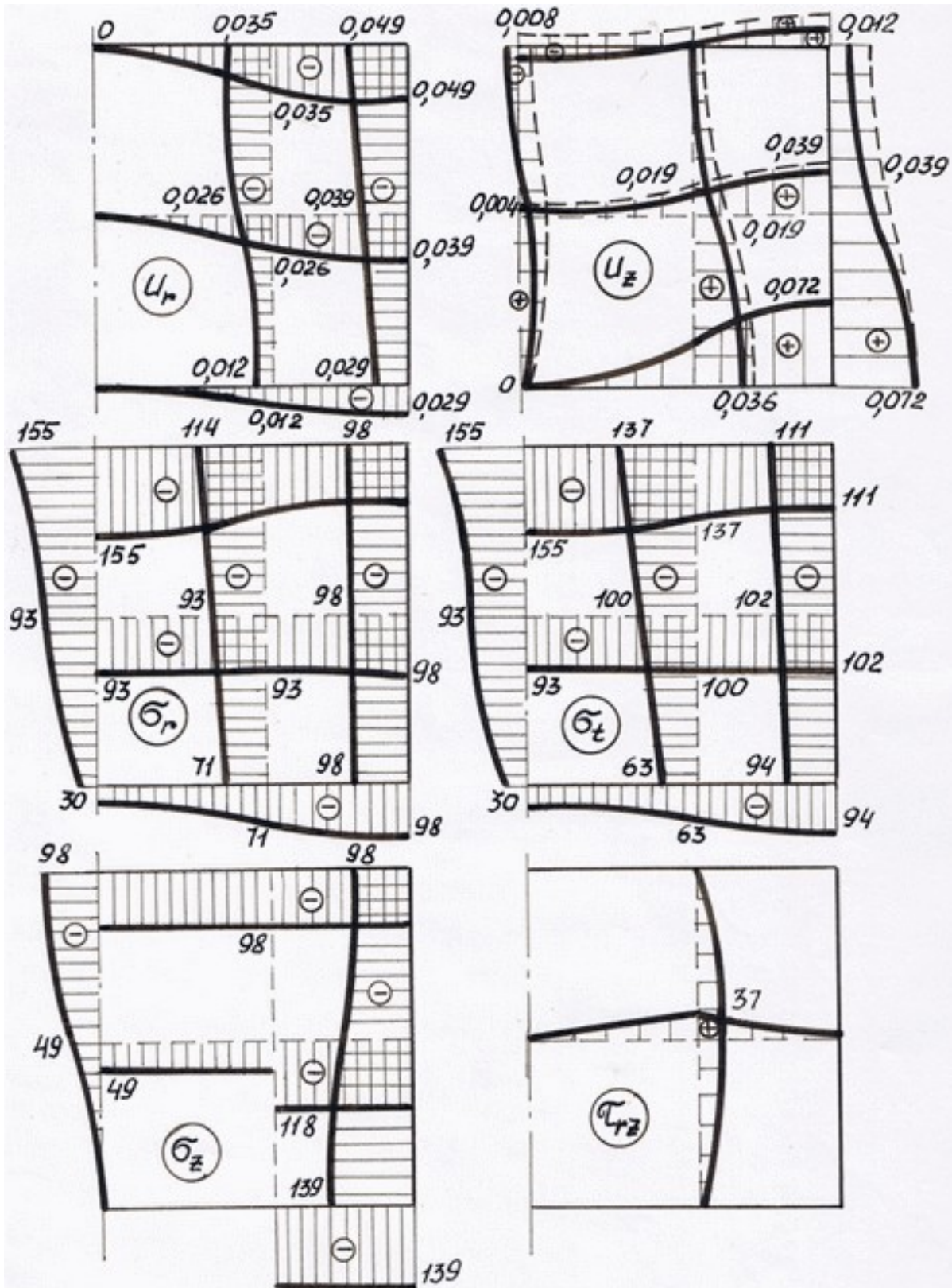
Рисунок 2.12. Эпюры перемещений в миллиметрах и напряжений в мегапаскалях, определённые по формулам (2.80) – (2.83), в сечениях z = 0, z = h/2, z = h, r = 0, r = a_1, r = a именно существенно трёхмерного сплошного цилиндрического тела, в частности светопрозрачного элемента, размерами a_1 = 30 мм, a = 55 мм, h = 60 мм из стекла К8 при давлениях p = p_1 = 98 МПа.
